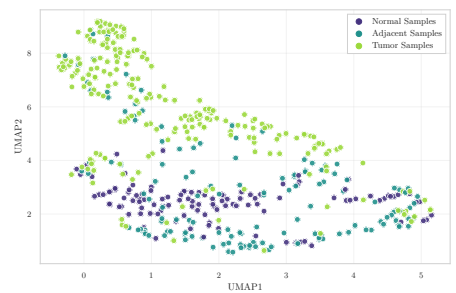
(c) UMAP
